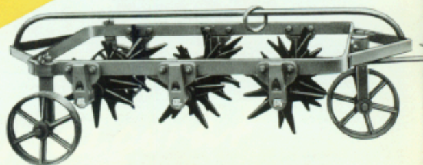
Abb. 3 Marke WKE 1 mit Fahrvorrichtung und Zugbügel für Kippflug
